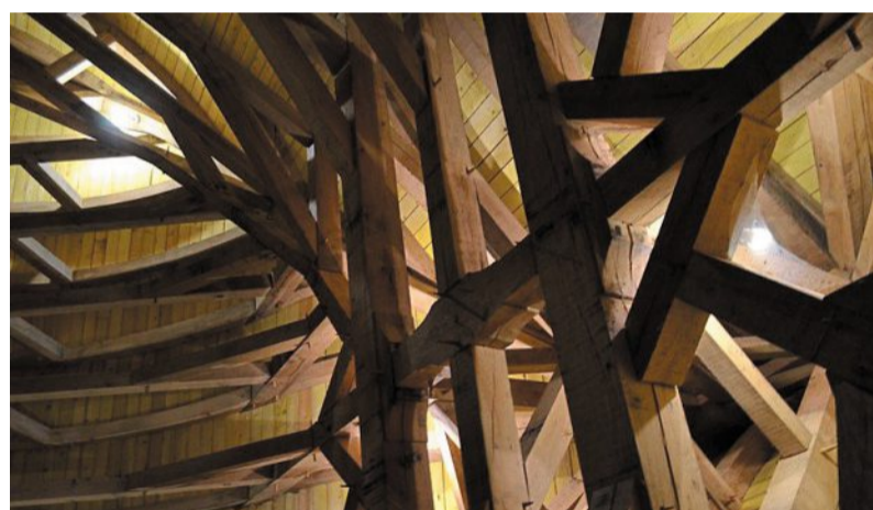
L'une des charpentes du manoir entièrement refaite à l'ancienne, sans aucun clou ni vis, seulement du chêne et des chevilles en bois PHOTO : LE MAINE LIBRE
